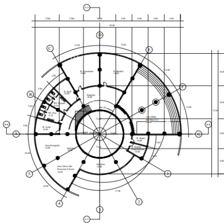
Gambar 13. Denah Lt.3 Sumber: Analisis penulis
