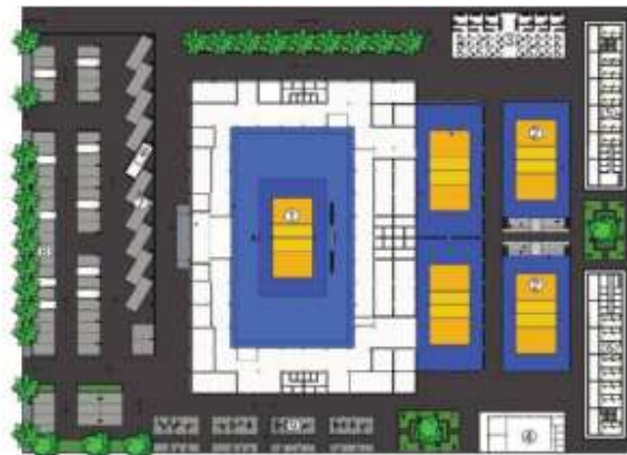
Gambar 14. Rencana Tapak
