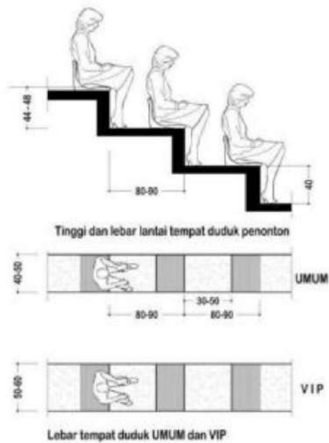
Gambar 3. Dimensi Kursi Tribun VIP Dan Umum Sumber: Permenpora, 2018
