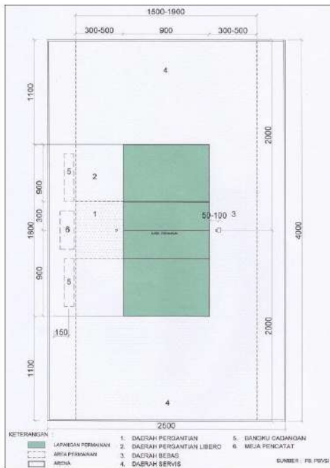
Gambar 1. Lapangan Pertandingan Bola Voli
