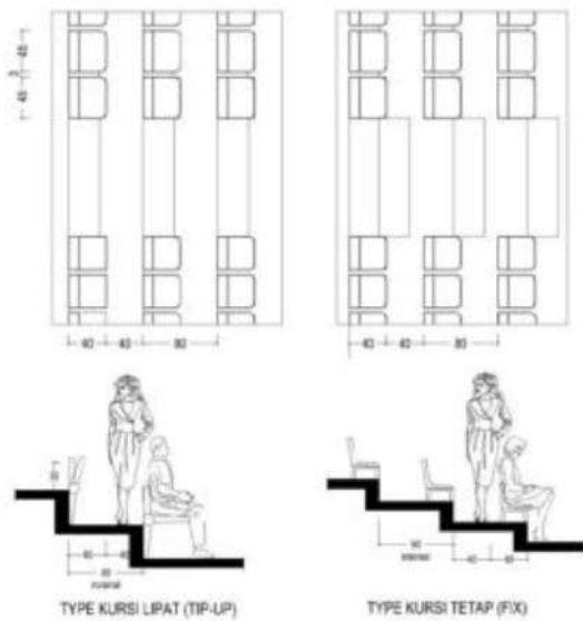
Gambar 4. Tipe Kursi Tribun Sumber: Permenpora, 2018
