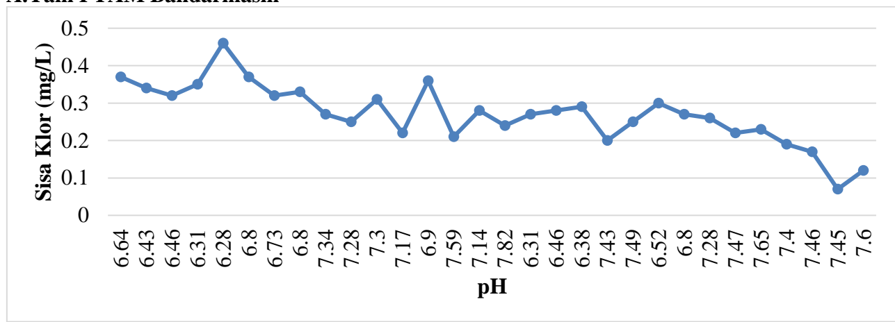
Gambar 3. Hubungan pH Terhadap Sisa Klor
