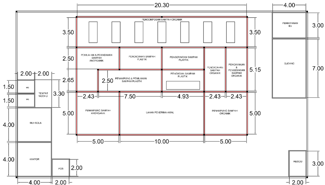
Gambar 5. Layout Denah Perencanaan TPS 3R Kecamatan Banjarbaru Utara
